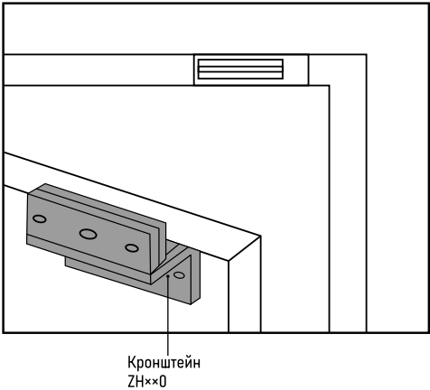
Рис. 1 Монтаж с помощью кронштейнов L- и Z-типов (LHx0 и ZHx0)
