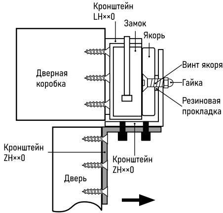
Рис. 1 Монтаж с помощью кронштейнов L- и Z-типов (LHx0 и ZHx0)
