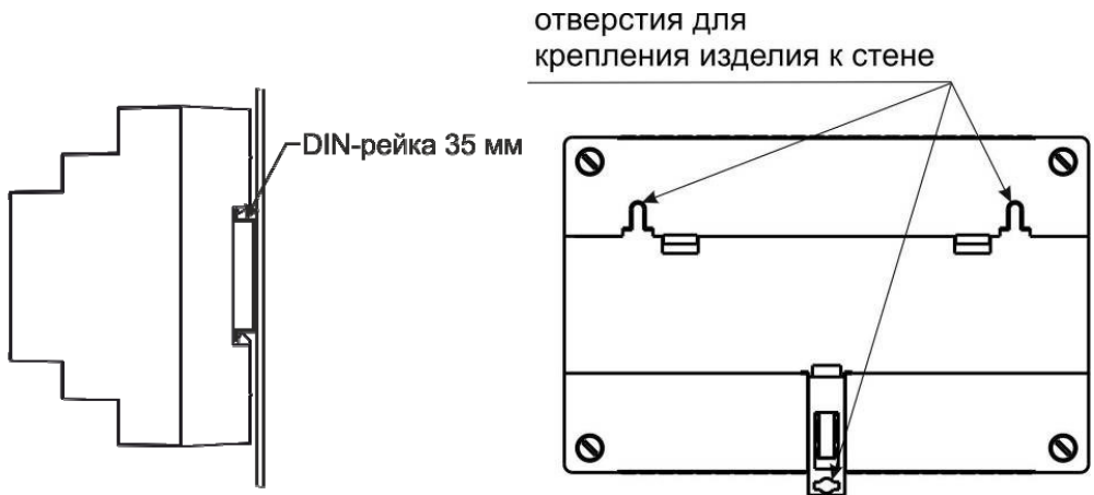
Рисунок 1 - Крепление изделия
