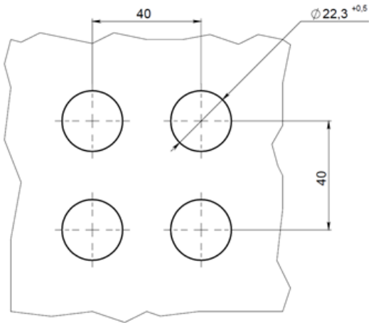
Монтажные размеры
