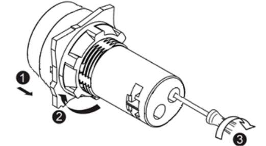
Монтаж зуммеров
