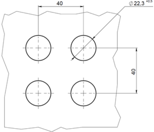
Монтажные размеры Рисунок 1 – Последовательность монтажа зуммеров
