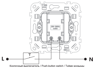
Рисунок 1 – Электрические схема звонка / Figure 1 – Electrical circuit of the bell / 1-сурет – Электрлік қоңырау схемасы
