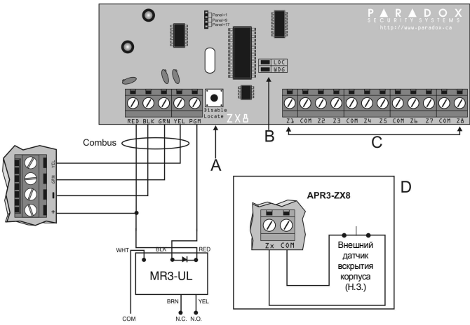
Картина 1: Подключение модуля APR-ZX8
